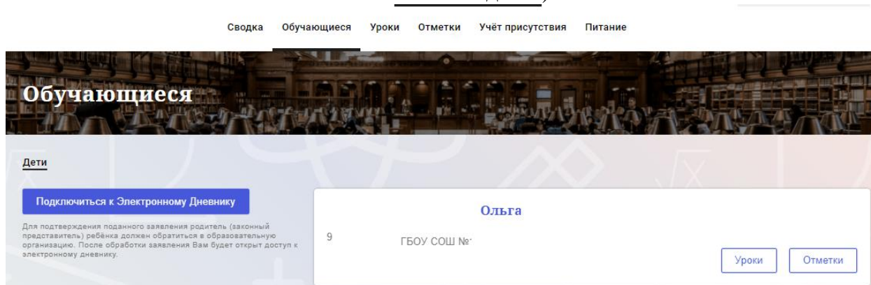
Рисунок 6 – Страница «Обучающиеся»
